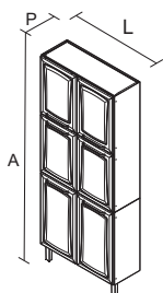
IPLD-80 PRODUTO MONTADO: A: 1,95 L: 0,80 P: 0,30 M
